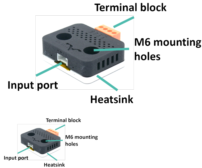
TicPWM module
